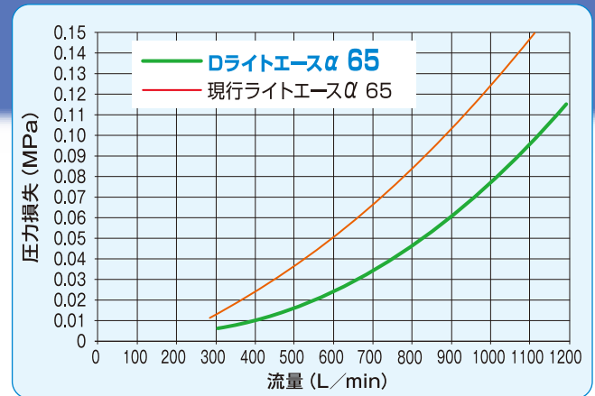
■65×20m 使用圧1.6MPaの圧力損失と流量の比較 (当社測定値)
