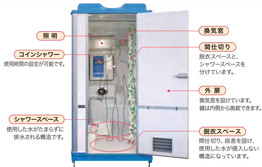
組立時外観
